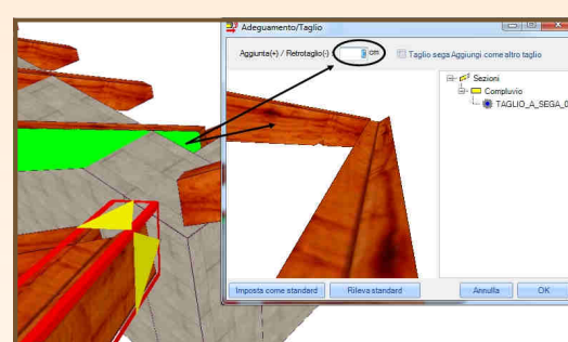
Coupe contrôlée des poutres selon références existantes
