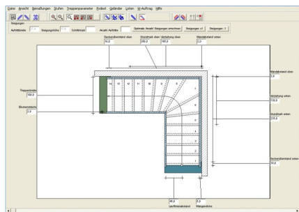
Vue en plan d'un escalier à un quartier tournant
